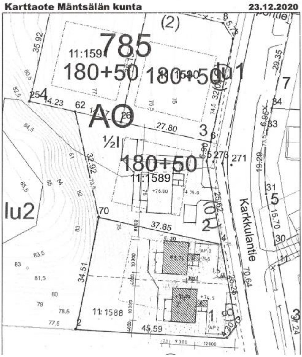
Liite 3: Rakennusluvan 21-0106-R asemapiirros
