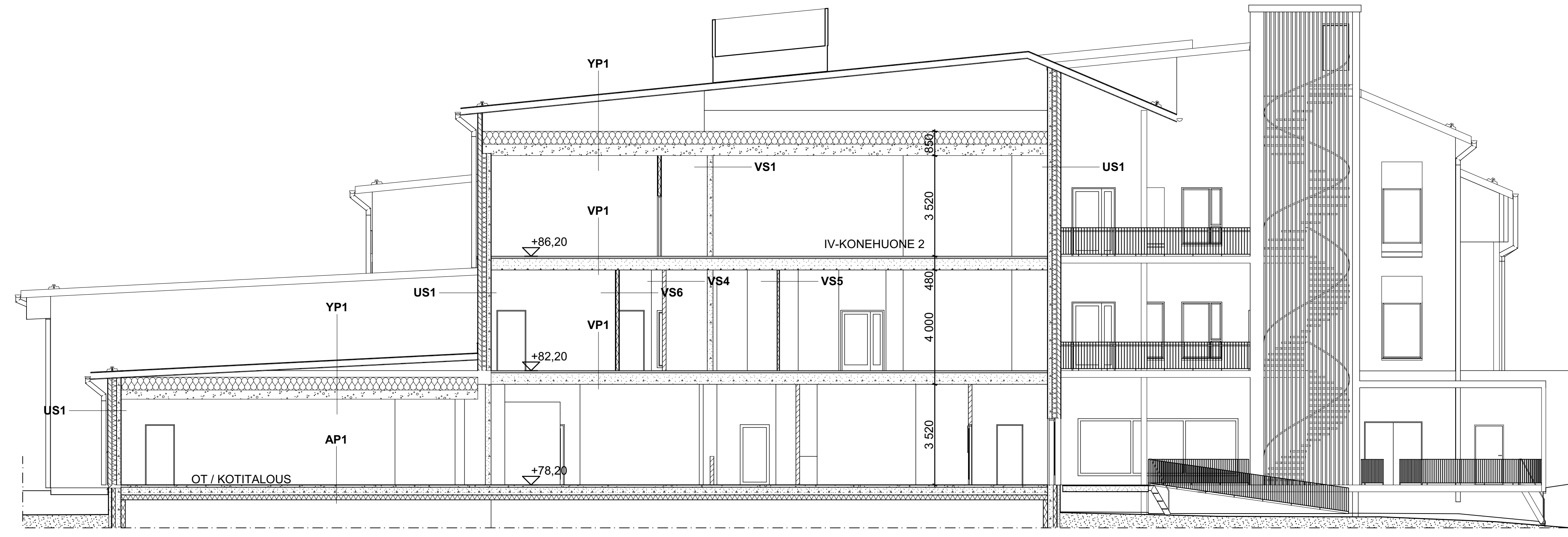
LEIKKAUS C-C
