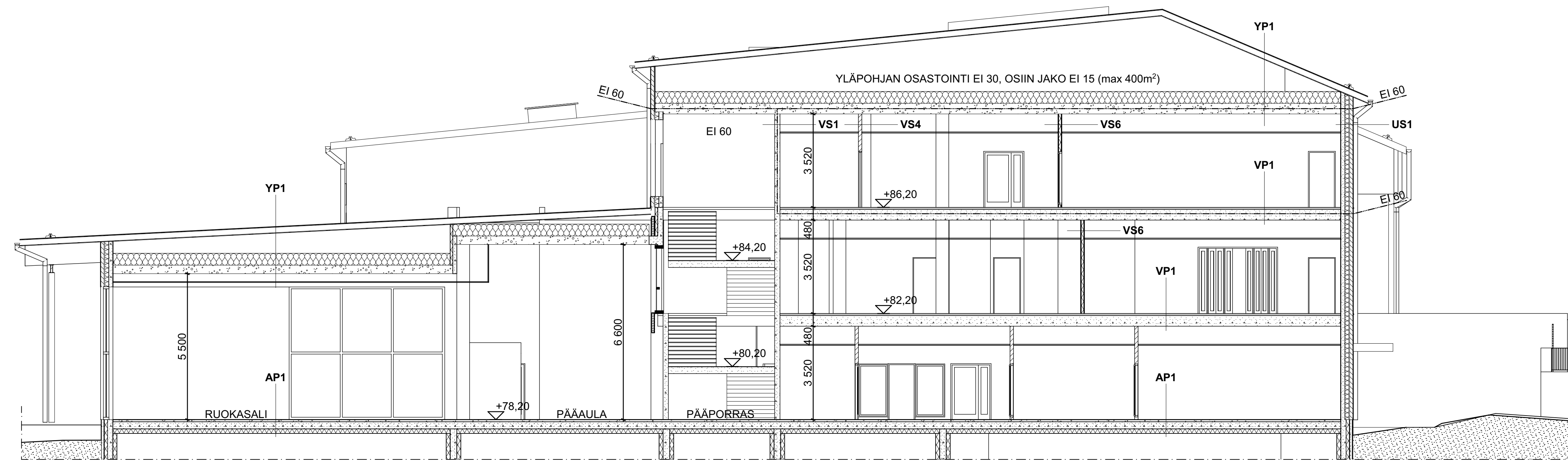
LEIKKAUS B-B
