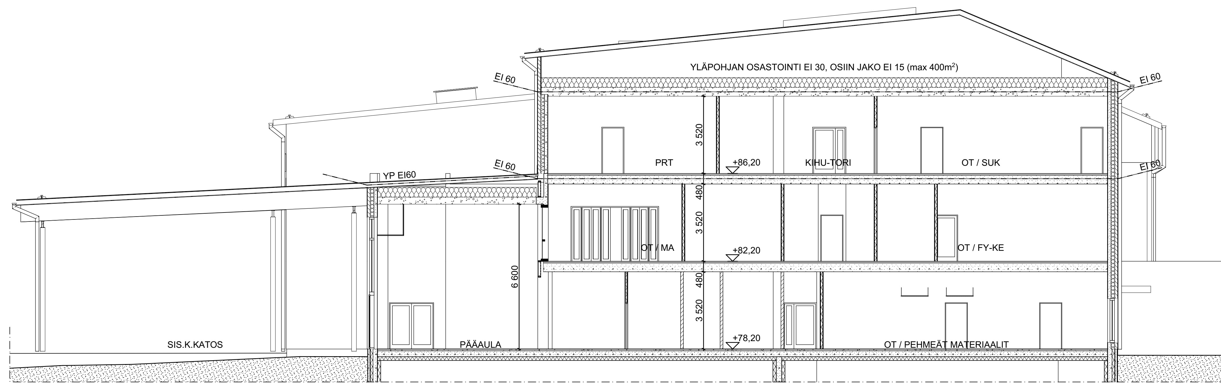
LEIKKAUS A-A
